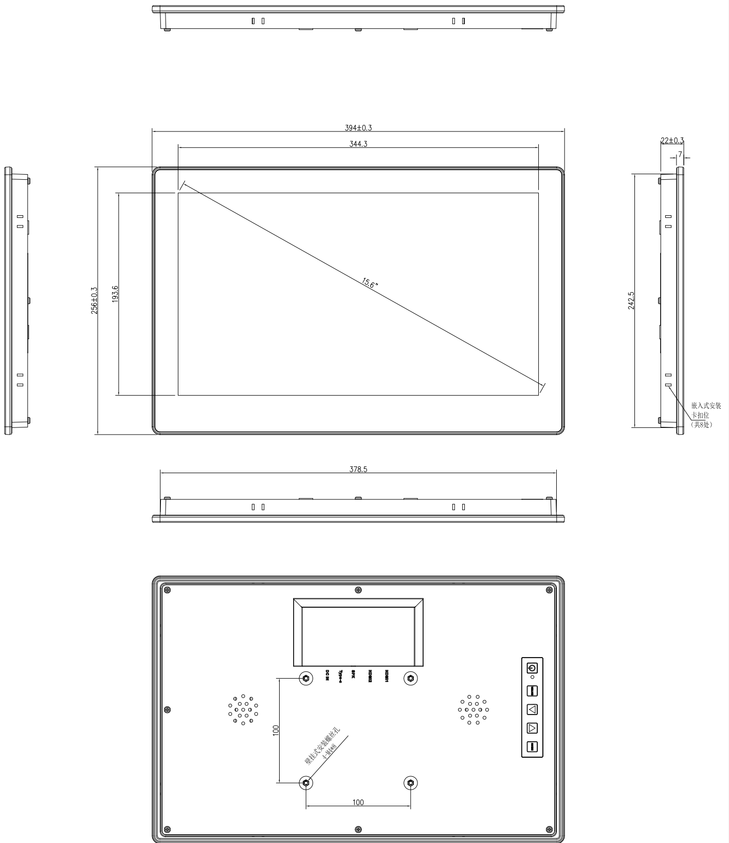
FPAD916显示器 嵌入式安装开孔尺寸：380*245MM
